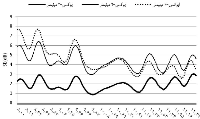
نمودار ۱- تغییرات مقادیر اثربخشی حفاظتی هر یک از سپرهای اپوکسی ساخته شده در باند بسامدی X
