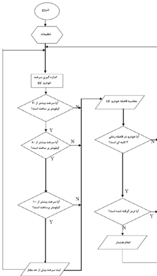
شکل ۲- فلوچارت سیستم FCW طراحی شده
