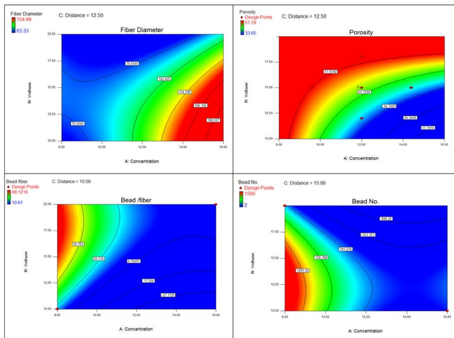
شکل ۱- پلات کنتوری از تاثیر همزمان غلظت و ولتاژ در فاصله الکتروریسی معین بر متغیرهای پاسخ
