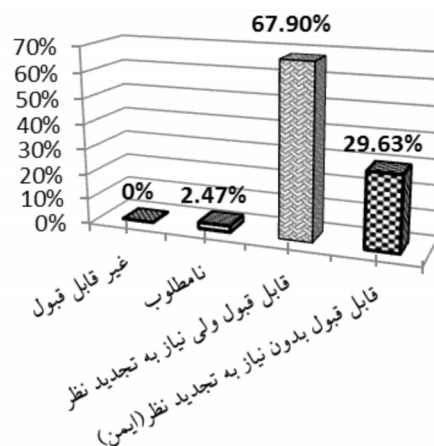
نمودار ۳ - نتایج نهایی سطح ریسک بعد از راهکار کنترلی
