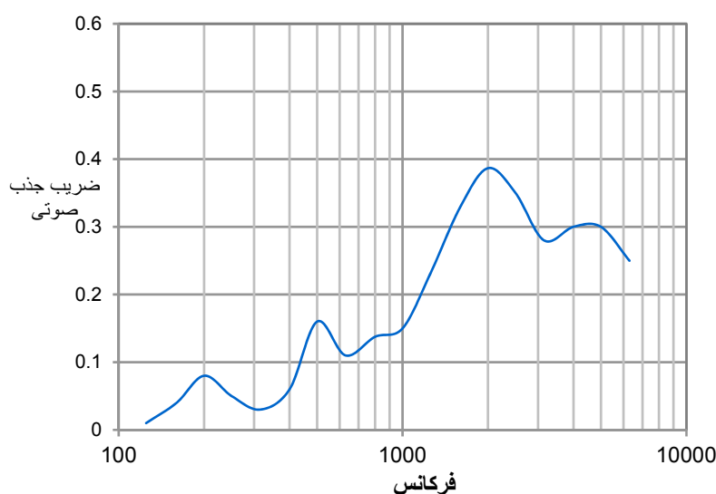
شکل ۵- نتایج اندازه‌گیری ضریب جذب فوم NBR-PVC با ضخامت ۲۱ میلیمتر
