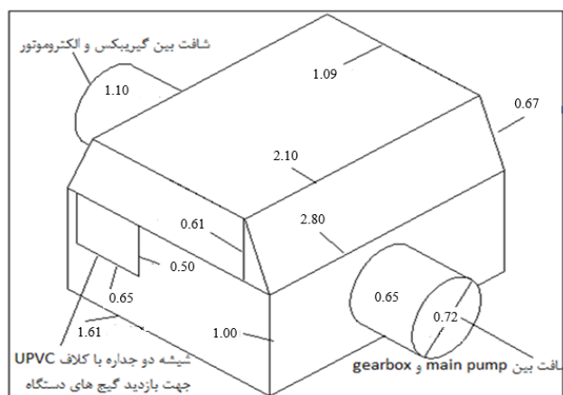
شکل ۳- نمای مونتاژ از اتاقک طراحی شده برای جعبه دنده (اندازه ها به متر)
