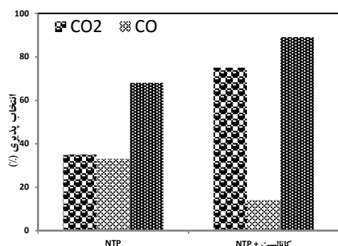
شکل ۷- انتخاب پذیری روش پلاسمای تنها و روش هیبریدی به \text{CO}_2 و \text{CO} در انرژی ورودی ویژه ۱۰۰۰ ژول بر لیتر (غلظت آلاینده ها ۳۰۰ ppm).
