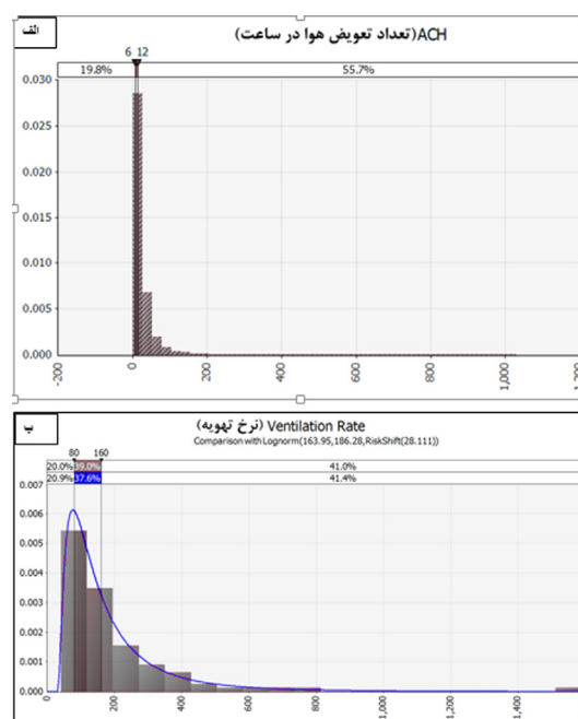
شکل ۴- درصد مقادیر استاندارد الف) ACH و ب) نرخ تهویه بر حسب لیتر بر ثانیه برای هر نفر در بخش‌های هوابرد
