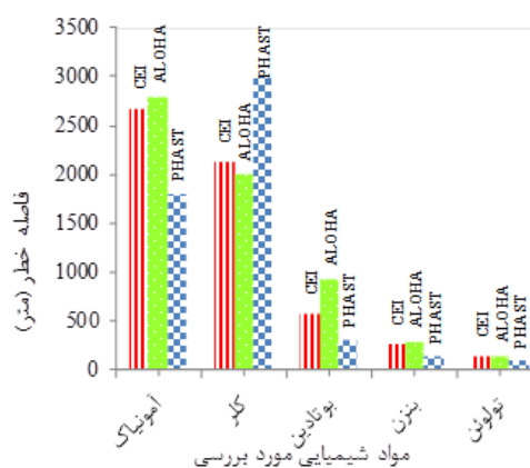
نمودار ۱۱- مقایسه فواصل خطر تعیین شده توسط نرم‌افزارهای ALOHA و PHAST و شاخص CEI براساس معیار ERPG-3 برای مواد شیمیایی مورد بررسی
