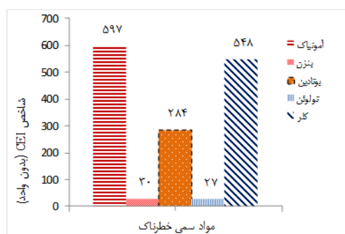
نمودار ۳- مقادیر شاخص CEI برای مواد سمی مورد مطالعه در ناوگان حمل‌ونقل جاده‌ای مواد خطرناک
