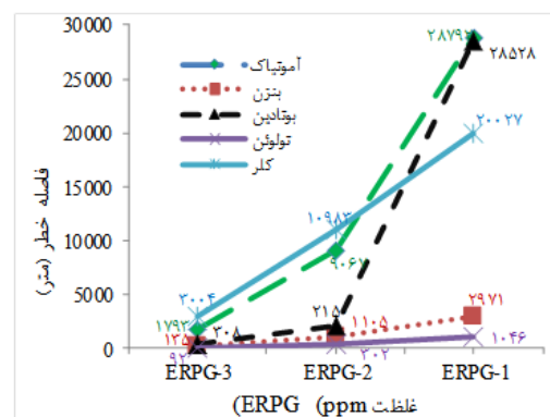
نمودار ۵- پیش بینی فاصله خطر حادثه شکافت کامل تانکرهای حامل مواد سمی براساس غلظت های ERPG توسط نرم افزار PHAST
