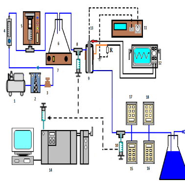
شکل ۱- شماتیک مجموعه آزمایشی مورد استفاده
