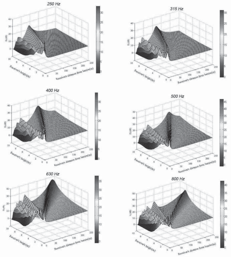
شکل ۳- نمودار سطحی افت صدا در فرکانس های ۱/۳ اکتاو باند بین ۲۵۰ تا ۸۰۰ هر تدر ۲۵۰۰ گیرنده در میدان وسیعی پشت مانع مرجع
