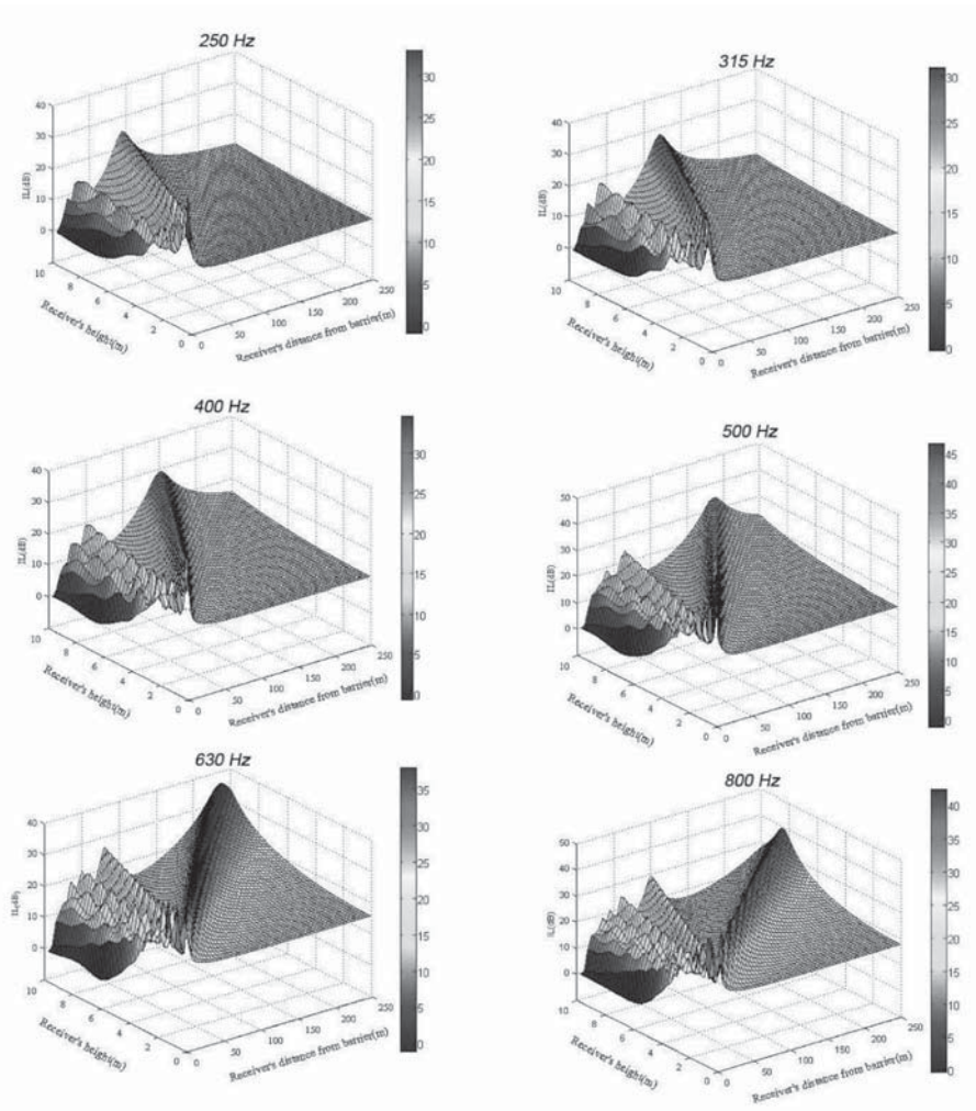
شکل ۳- نمودار سطحی افت صدا در فرکانس های ۱۱/۳ اکتاو باند بین ۲۵۰ تا ۸۰۰ هر تدر ۲۵۰۰ گیرنده در میدان وسیعی پشت مانع مرجع
