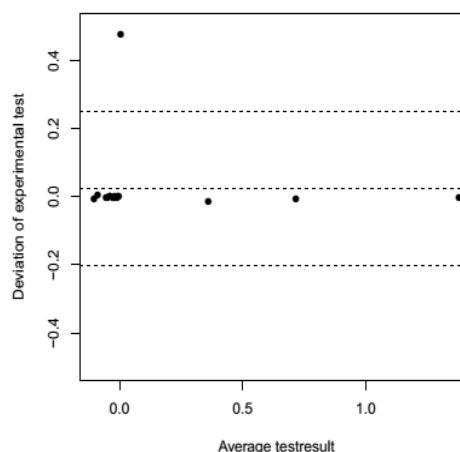
شکل ۵- نمودار بلند-آلتمن برای تطابق درصد‌های اختلاف فشار کل اندازه‌گیری شده و محاسبه شده در یک سیستم دارای سه هود
