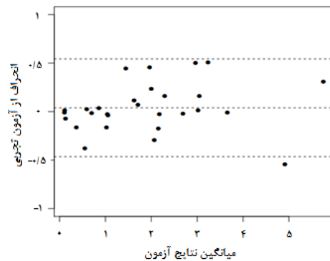
نمودار ۱- توافق دو روش UV و FT-IR در تعیین مقدار روغن‌های معدنی با آزمون آماری بلند و آلتمن
