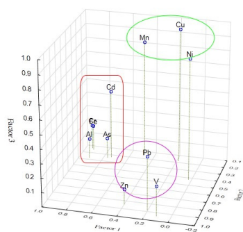
شکل ۴- نمودار تعیین تعداد منابع محتمل انتشار عناصر موجود در ذرات برحسب مقادیر Eigenvalues در مجتمع پردازش و دفع آرادکوه الف
