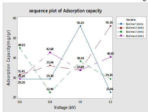
شکل ۴- تأثیر افزایش زمان مواجهه با پلازما بر حسب تابعی از ولتاژ اعمال شده بر فرایند اصلاح
