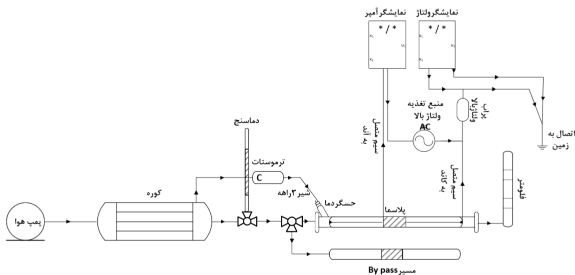
شکل ۱- سیستم آزمایشگاهی اصلاح کربن فعال با پلاسما
