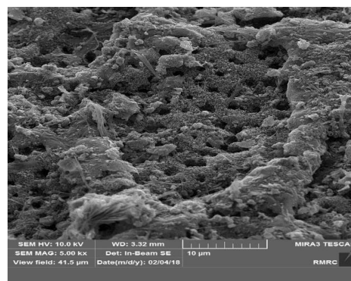
شکل ۹- Fe-SEM/گرانول کربن فعال اصلاح نشده بزرگنمایی ۵۰۰۰ (مقیاس \mu\text{m} )
