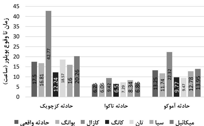
شکل ۳- مقایسه نتایج پیش‌بینی مدل‌های تجربی با حوادث واقعی
