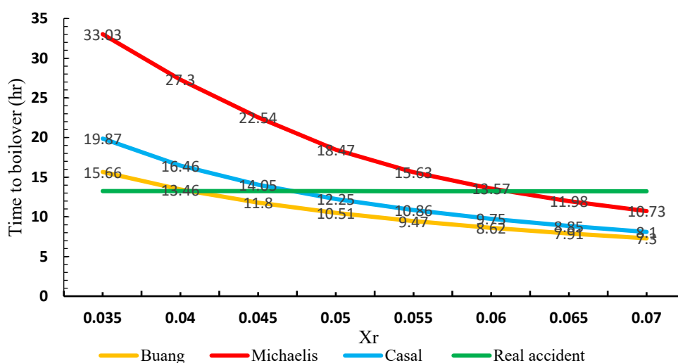
شکل ۴- زمان وقوع Boilover حادثه پالایشگاه آموکو برای دامنه ای از کسر حرارتی بازتابی
