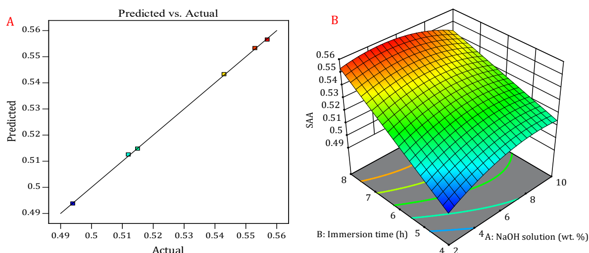
شکل ۳- الف) مقادیر واقعی در مقابل مقدار پیش بینی شده مدل (ب) نمای سه بعدی تأثیر متغیرهای اصلی بر AAS در فرآیند اصلاح آکالینی
