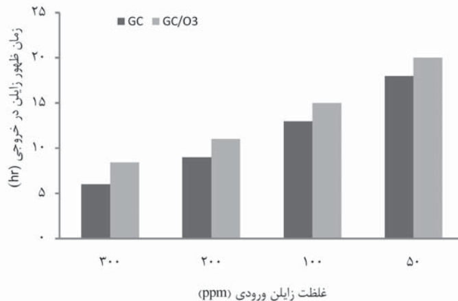
شکل ۲- مقایسه زمان ظهور زایلن در سیستم کربن فعال (GC) با فرایند ازن زنی کاتالیزوری (GC/O3) در غلظتهای مختلف
