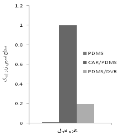
شکل ۱- میزان نسبی بازیافت ۲-کلروفنول از روی فیبرهای PDMS 100μm، CAR/PDMS 75μm و PDMS/DVB 65 در حالت تماس یافته خارج از غلاف
