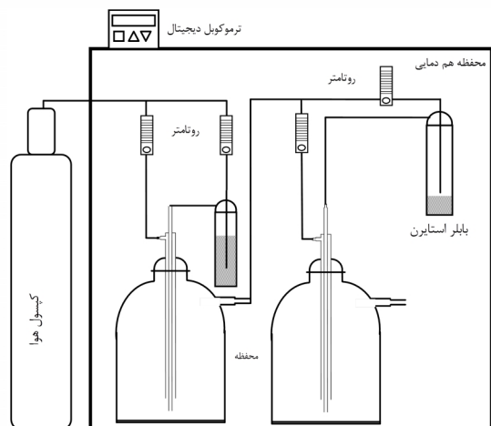
شکل ۲- مدار سیستم غلظت ساز بخارات توسط بایلر
