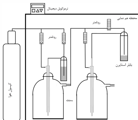
شکل ۲- مدار سیستم غلظت ساز بخارات توسط بایلر
