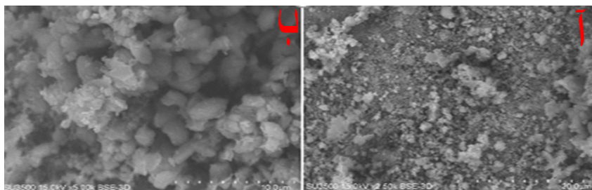
شکل ۳- تصاویر SEM بستر زئولیت Y آغشته به نانو ذرات TiO 2 (A) بزرگنمایی ۲۵۰۰ (ب) بزرگنمایی ۵۰۰۰
