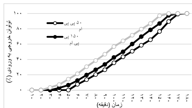
نمودار ۳- بررسی ظرفیت جذب بستر دی: ۱ لیتر بر دقیقه، دما: ۲۳±۲، غلظت: ۵۰، ۱۵۰، ۳۰۰ پی پی ام، رطوبت: ۴۰٪
