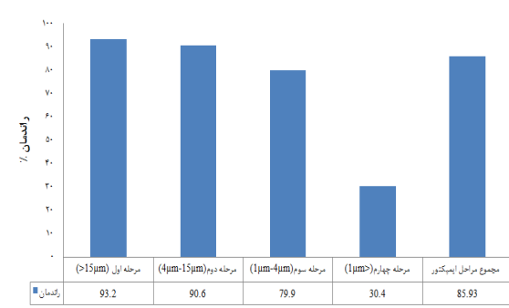
نمودار ۲. کارایی حذف سایزهای مختلف آلاینده توسط پالایشگر
