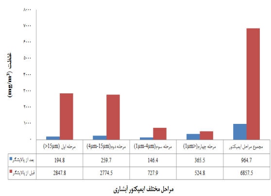
نمودار ۱. مقایسه میانگین غلظت گردوغبار قبل و بعد از پالایشگر در بخش‌های مختلف نمونه‌بردار برخوری چهار مرحله‌ای
