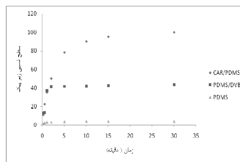
شکل ۸- استخراج ۲-کلروفنول با استفاده از فیبرهای 100 \mu m PDMS، 65 \mu m PDMS/DVB و 75 \mu m CAR/PDMS در حالت تماس یافته خارج از غلاف
