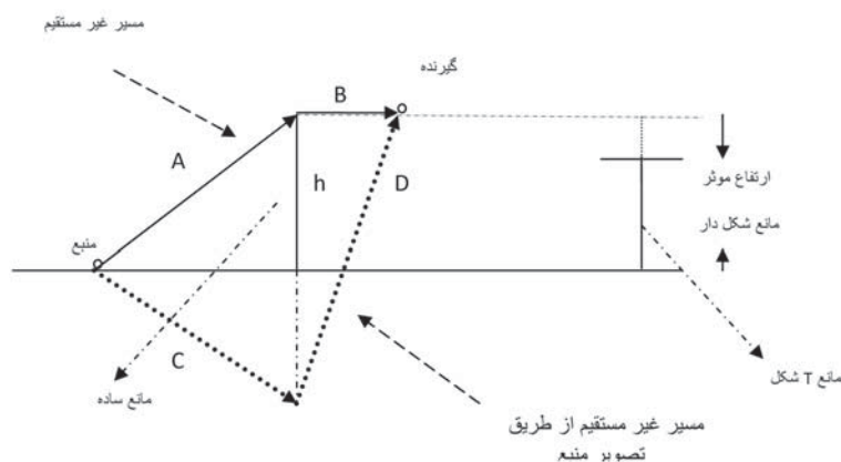
شکل ۱- شکل هندسی امواج غیر مستقیم مانع و تصویر مطابق با ارتفاع مؤثر مانع T شکل
