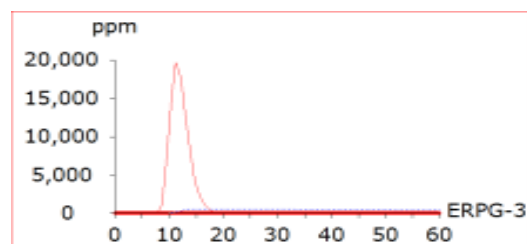
نمودار ۳- نمودار غلظت بر مبنای معیار ERPG برای انتشار گاز CK
