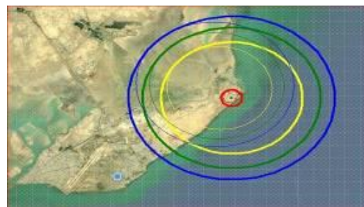
شکل ۳- کنتور نشت عمدی AC در مرکز نیروگاه هسته‌ای بوشهر (مساحت منطقه قرمز، زرد و سبز به ترتیب ۳/۵۶۷۸۲e+۷۰۰۷۰۲۰۰۷ و ۵/۸۱۶۴۲e+۰۰۷ مترمربع می‌باشد).
