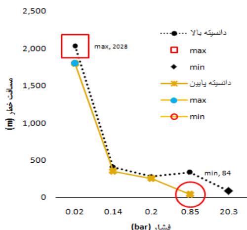
نمودار ۱- مسافت خطر انفجار در دانشیه بالا و پایین
