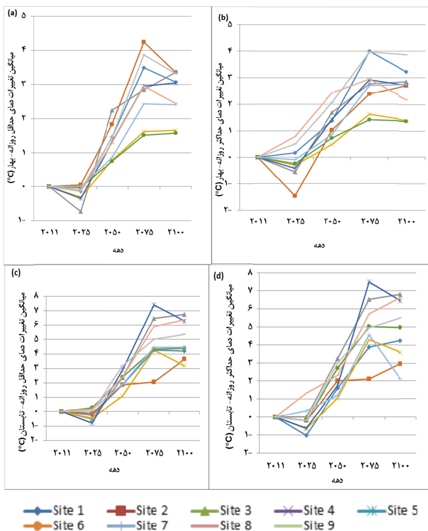
شکل ۳- میانگین اختلاف حداقل و حداکثر روزانه در دهه های آتی در مقایسه با شرایط کنونی (بر اساس داده های هوا شناسی قابل استفاده سال ۲۰۱۱). (a) میانگین تغییرات دمایی حداقل روزانه در مقایسه با شرایط کنونی در فصل بهار (b) میانگین تغییرات دمایی حداقل روزانه در مقایسه با شرایط کنونی در فصل بهار (c) میانگین تغییرات دمایی حداقل روزانه در مقایسه با شرایط کنونی در فصل تابستان (d) میانگین تغییرات دمایی حداقل روزانه در مقایسه با شرایط کنونی در فصل تابستان
