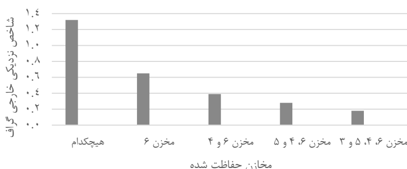
نمودار ۲. تأثیر ضدحریق‌سازی مخازن بحرانی گسترش‌دهنده‌ی سناریوهای زنجیره‌ای بر کاهش آسیب‌پذیری مجموعه مخازن.
