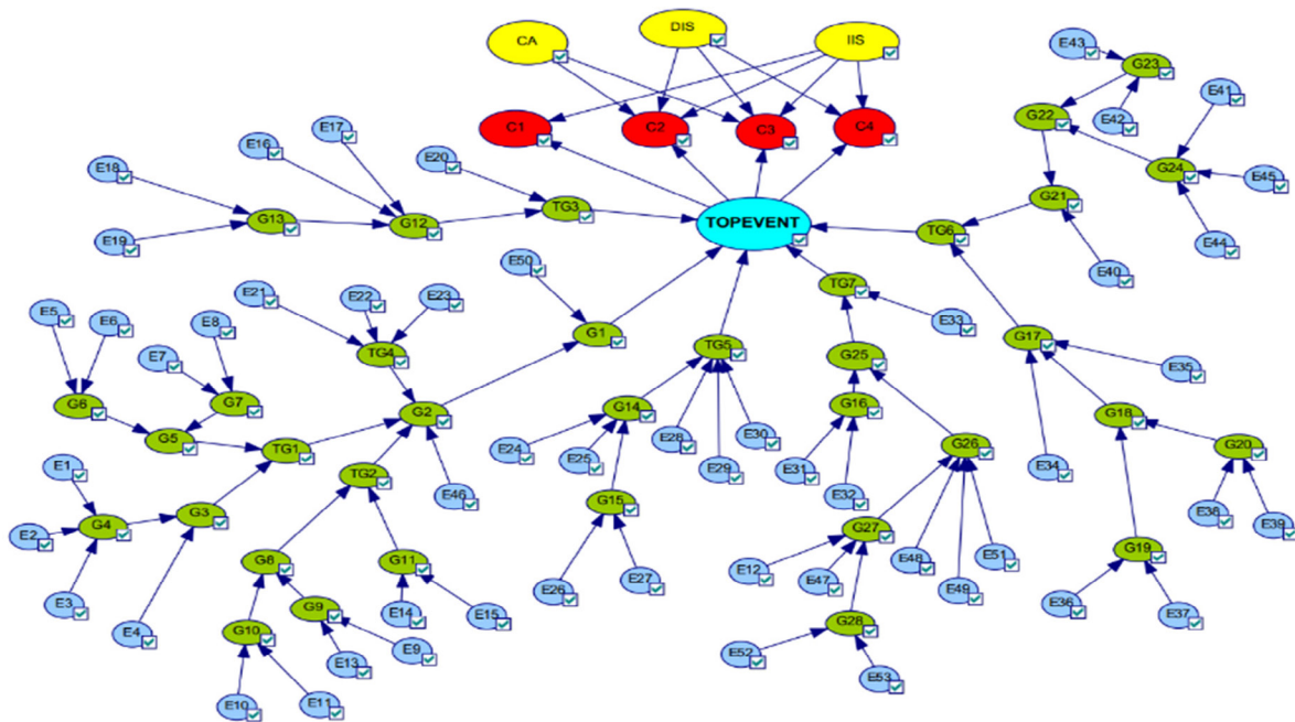
شکل ۵. شبکه بیزین مخزن LPG
