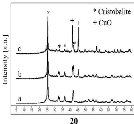
شکل ۱- الگوهای XRD دیاتومیت خام و کاتالیست تهیه شده با غلظت ۱wt% و ۴wt% نانوذرات اکسید مس بعد از کلسیناسیون در دمای 450^{\circ}\text{C} : (a) دیاتومیت خام، (b) کاتالیست با غلظت ۱ درصد وزنی CuO و (c) کاتالیست با غلظت ۴ درصد وزنی CuO.
