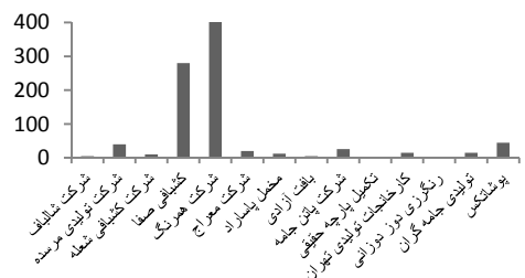
نمودار ۲- میزان اکسیژن مورد نیاز بیولوژیکی (BOD) صنایع مورد بررسی
