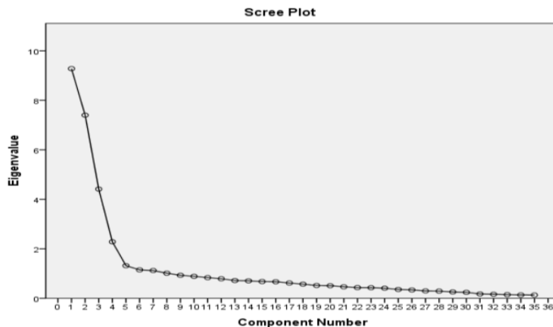
نمودار ۱- نمودار اسکرین (مقادیر ارزش‌های ویژه) پرسشنامه‌ی ۳۵ سؤالی فرهنگ ایمنی
