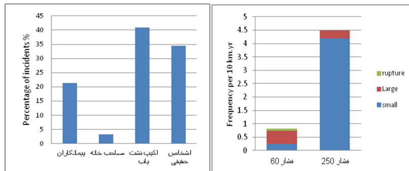
شکل ۶- ارتباط بین سایز نشت و فشار شبکه توزیع شکل ۷- نحوه کشف و گزارش نشت
