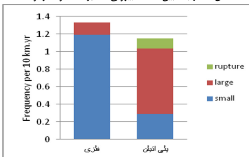
شکل ۱۰- ارتباط بین جنس شبکه و سایز نشت
