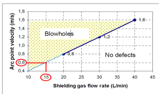
شکل ۱- نسبت سرعت در نقطه قوس و میزان جریان حجمی گاز محافظ - مرزی که نقص‌های جوشکاری رخ می‌دهد (مطالعه ایواساکی و همکاران)
