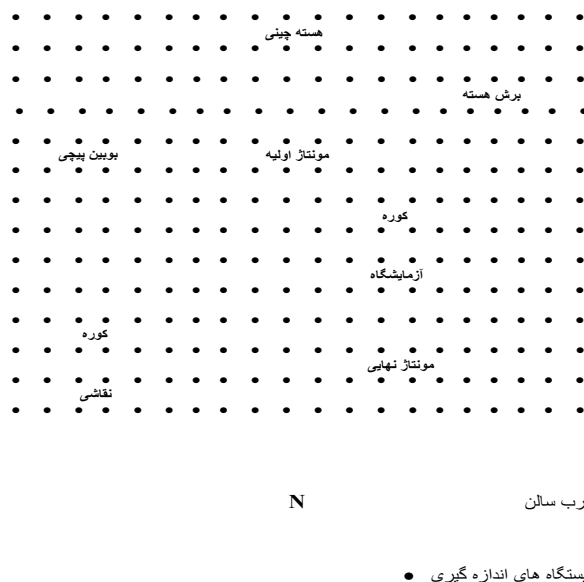
شکل ۱- نیمرخ افقی سالن مونتاز و موقعیت ایستگاه‌های اندازه‌گیری در ارتفاع سطح کار
