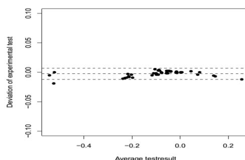
شکل ۳- نمودار بلند-آلتمن برای تطابق درصدی اختلاف فشار استاتیکی اندازه‌گیری شده و محاسبه شده در یک سیستم دارای سه هود
