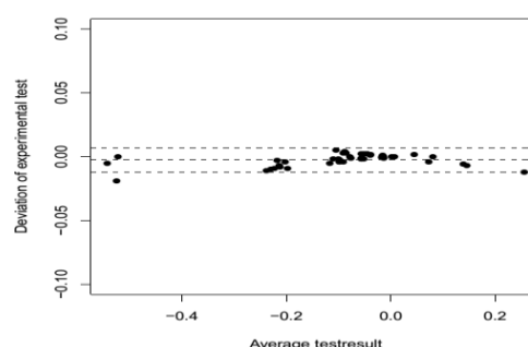
شکل ۳- نمودار بلند-آلتمن برای تطابق درصدی اختلاف فشار استاتیکی اندازه‌گیری شده و محاسبه شده در یک سیستم دارای سه هود
