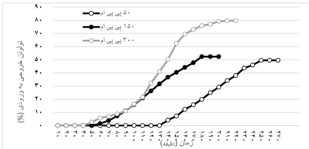
نمودار ۱- حذف فتوکاتالیستی تولون. دبی: ۱ لیتر بر دقیقه، دما: 22 \pm 2 ، غلظت: ۵۰، ۱۵۰، ۳۰۰ پی پی ام، رطوبت: ۴۰٪
