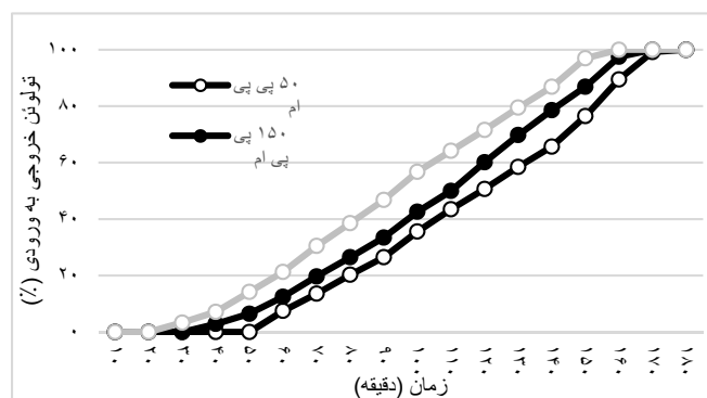
نمودار ۳- بررسی ظرفیت جذب بستر دی: ۱ لیتر بر دقیقه، دما: 23 \pm 2 ، غلظت: ۵۰، ۱۵۰، ۳۰۰ پی پی ام، رطوبت: ۴۰٪
