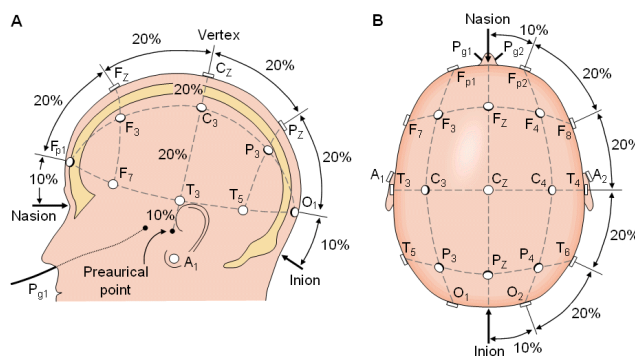
شکل ۳- نحوه چیدمان الکترودها در سیستم بین المللی ۱۰-۲۰ [۲۷]
