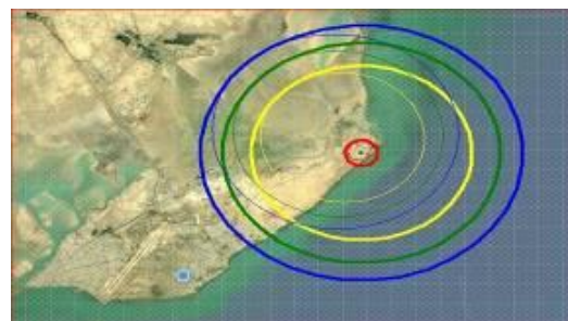
شکل ۳- کنتور نشت عمدی AC در مرکز نیروگاه هسته‌ای بوشهر (مساحت منطقه قرمز، زرد و سبز به ترتیب 7.072,007 \times 10^3 / 56782e و 5.81642e+007 مترمربع می‌باشد).
