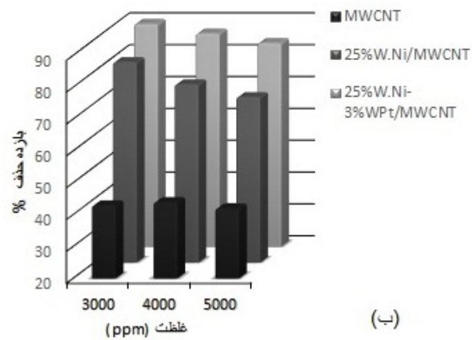
شکل ۶. بازده حذف کاتالیستی در غلظت های ۳۰۰۰-۴۰۰۰-۵۰۰۰ ppm و دمای ۲۵۰ و سرعت های فضایی (الف) ۱۵۰۰/hr (ب) ۲۰۰۰/hr.
