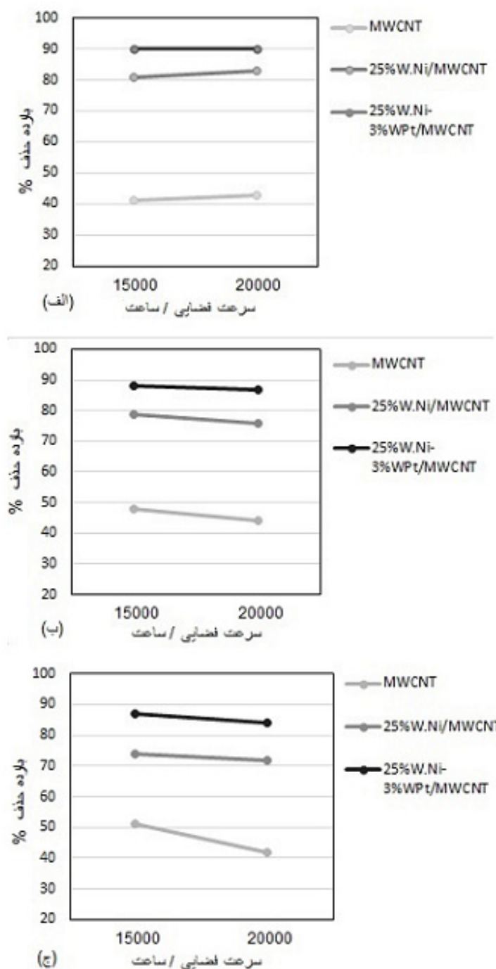
شکل ۷. بازده حذف کاتالیستی در سرعت های فضایی 15000-20000 \text{ hr}^{-1} ، دمای 250^{\circ}C و غلظت های (الف) 3000 \text{ ppm} (ب) 4000 \text{ ppm} (ج) 5000 \text{ ppm} .
