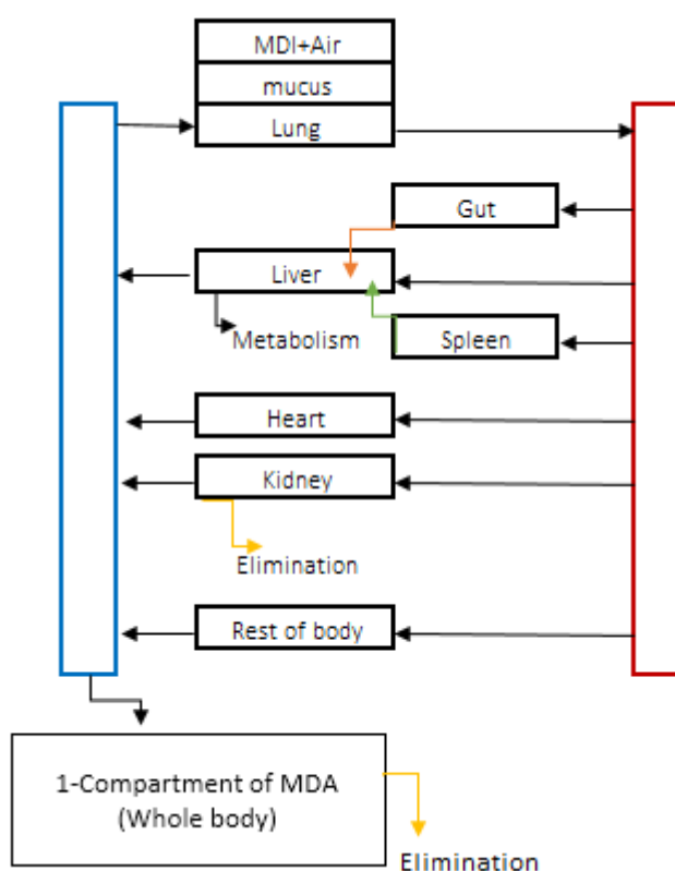
شکل ۱. ساختار کلی مدل برای پیش بینی دزیمتری بیومارکر MDI، کوپه lung نمایانگر بافت ریه، gut: دستگاه گوارش، liver: کبد، spleen، طحال، heart: قلب، kidney: کلیه و کوپه Rest of body شامل پوست، استخوان، چربی، مغز و ماهیچه است.
