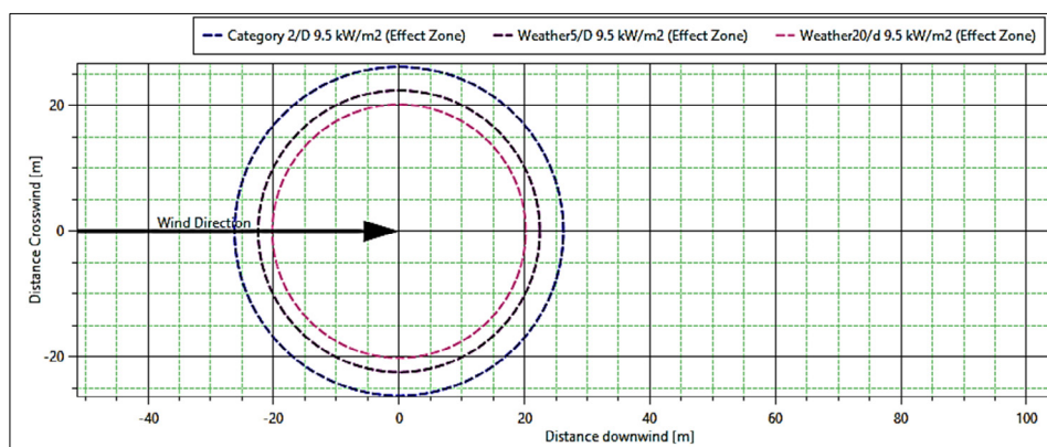
شکل ۴. شعاع تحت تأثیر تشعشعات آتش فورانی در حادثه نشتی تانکر بنزین
