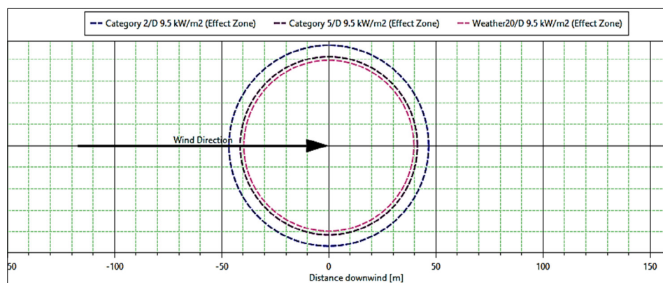
شکل ۶. شعاع تحت تأثیر تشعشعات ناشی از آتش فورانی در حادثه نشتی تانکر گاز مایع
