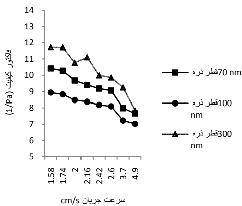
شکل ۷- فاکتور کیفیت (QF) صافی اولپا برای ذرات در گستره ۷۰، ۱۰۰ و ۳۰۰ نانومتر در سرعت جریان ۱.۵۸ تا 4.9 \text{ cm.s}^{-1}
